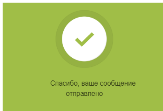
Рисунок 4 – заявка принята
